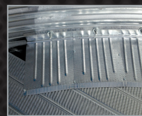
Y duct - any size
